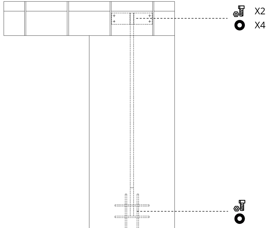
LONGHERONE Spar
