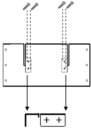
PIASTRE FISSAGGIO LIBRERIA Bookcase fixing plate
